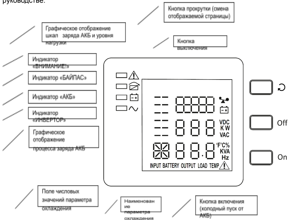
Рисунок 3 - ЖК—дисплей
