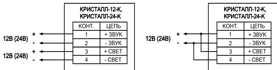
Рис.1. Схемы подключения.
