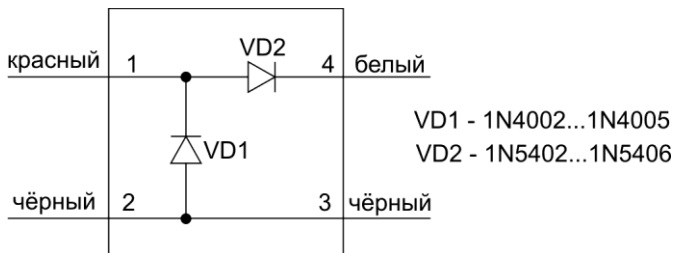
Рисунок 3. Схема модуля подключения нагрузки (МПН)
