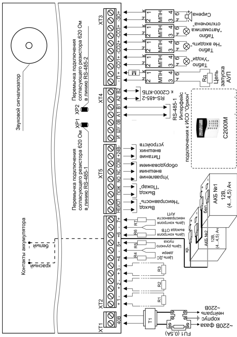
Рисунок 2. Схема внешних соединений блока
