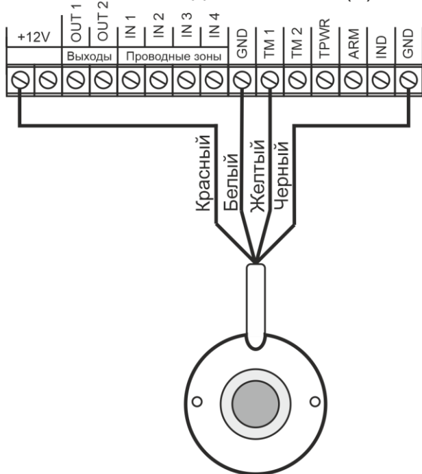
Клеммная колодка ИПРо - 7 (6)
