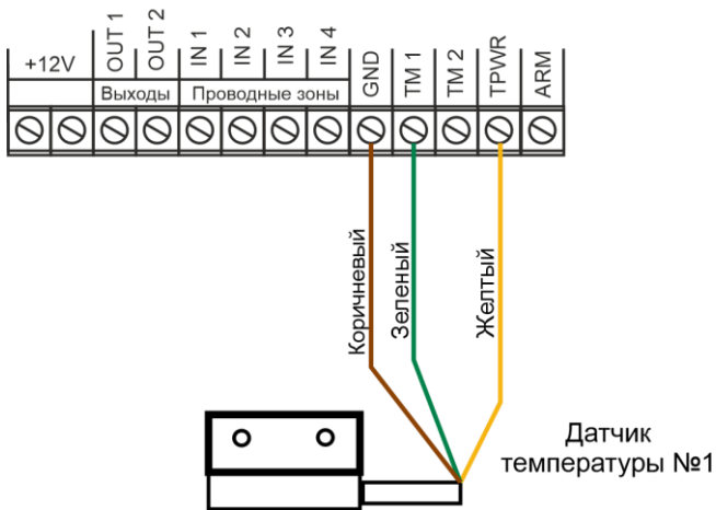
Клеммная колодка ИПРО - 7
