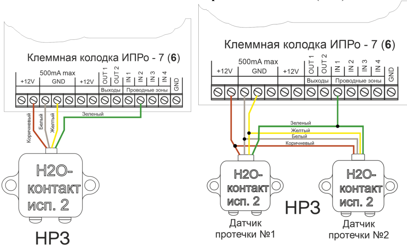
Подключение одного датчика
