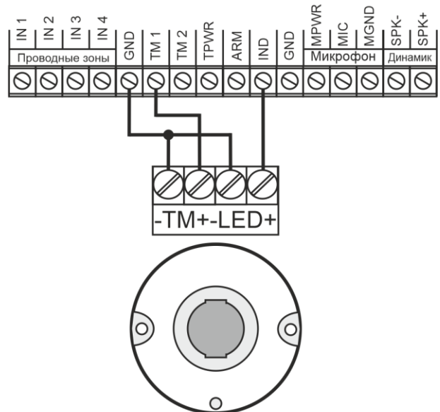
Клеммная колодка ИПРо - 7 (6)
