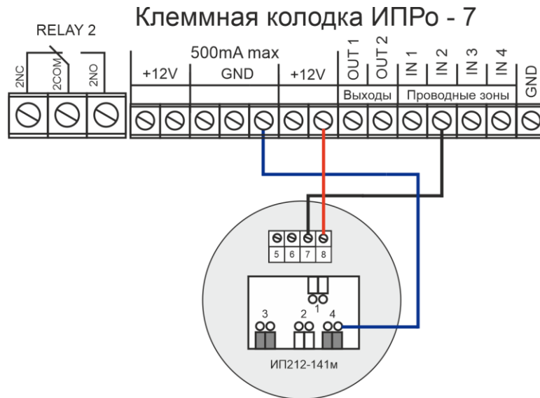
Подключение одного датчика
