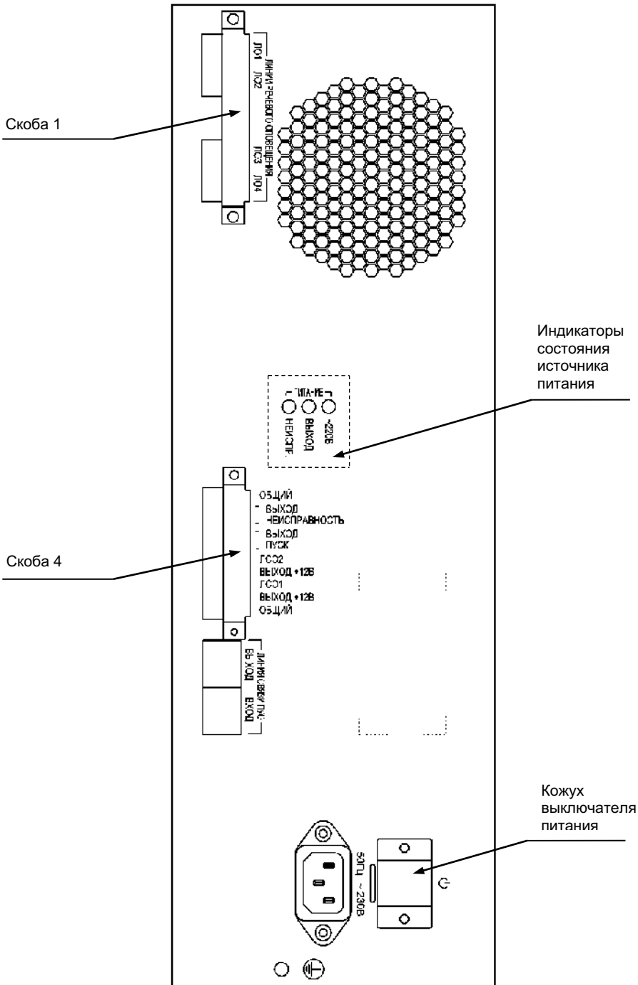
Рис.3 Внешний вид задней панели УМ
