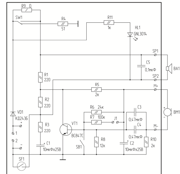
Схема электрическая принципиальная ТАП ЦИФРАЛ КМ-3
