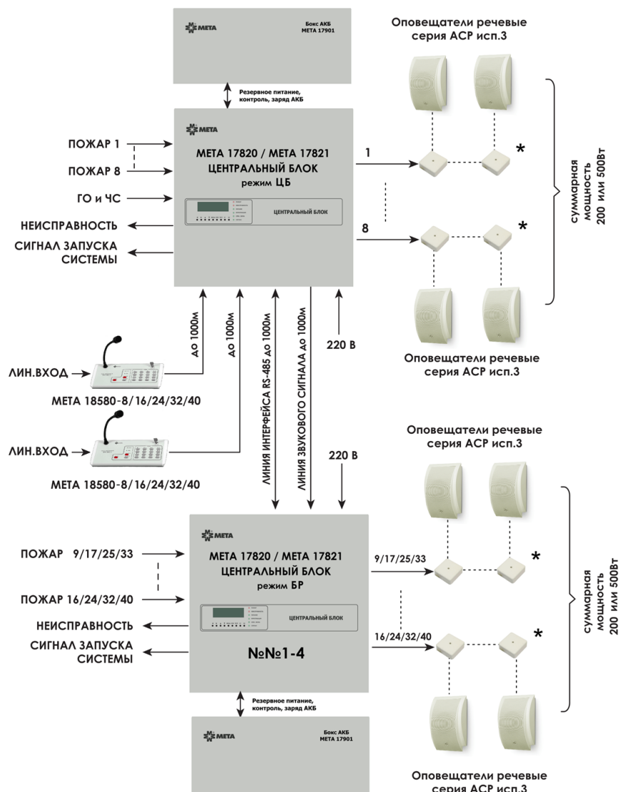
Рисунок 13. Структурная схема, построенная на базе ЦБ МЕТА 17820/17821.
