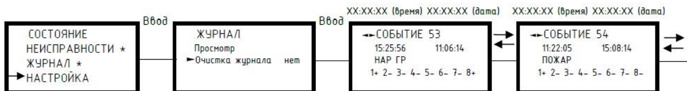
Рисунок 36. Журнал событий.
