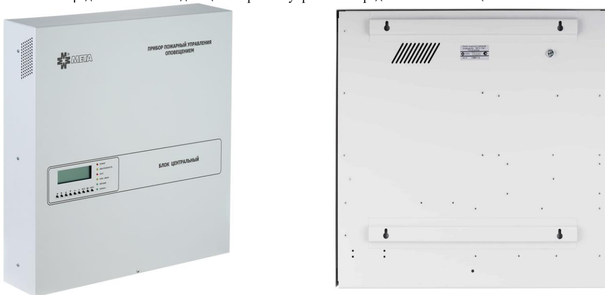
Рисунок 1. Внешний вид панели ЦБ МЕТА 17820/17821.
