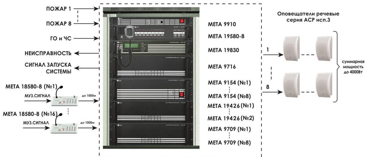
Рисунок 14. Структурная схема, построенная на базе ЦБ МЕТА 19830.
