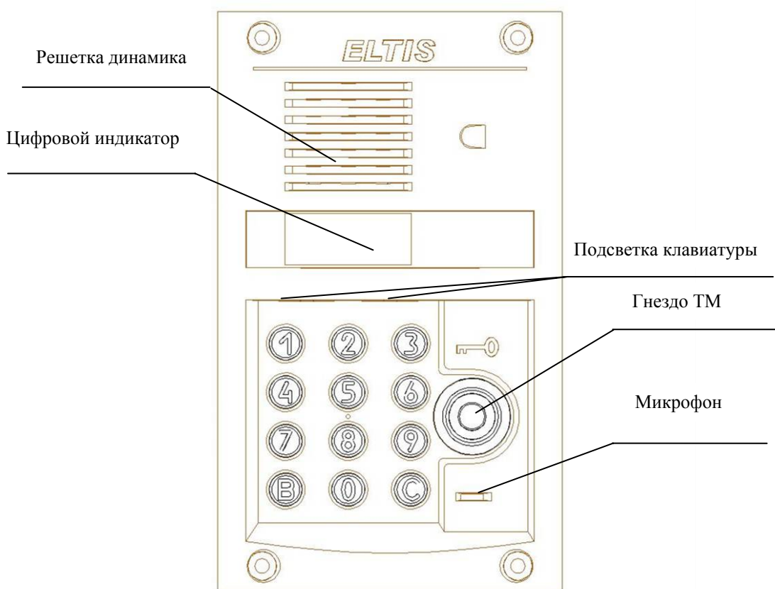
Рис.1 Внешний вид со стороны лицевой панели блока вызова DP420-TD22.
